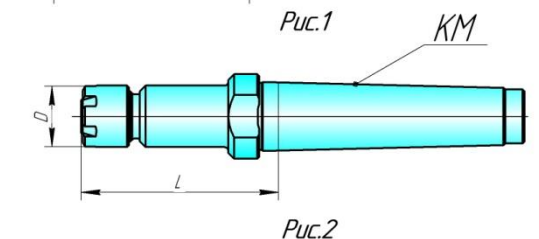
Цанговые патроны с цилиндрическим хвостовиком (рис.3)
