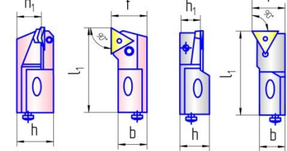
Рис.1-4 Система крепления P-рычагом Pic.1-4 Fastening system (P-Lever) Рис.5 Система крепления S-винтом Pic.5 Fastening system (S-screw)
