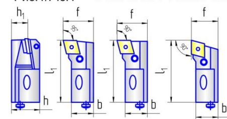
Рис.1-3 Система крепления P-рычагом Pic.1-3 Fastening system (P-Lever)
