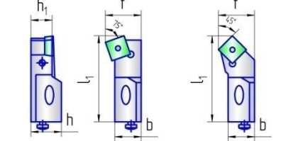
Рис.1-3 Система крепления P-рычагом Pic.1-3 Fastening system (P-Lever) Рис.4-5 Система крепления S-винтом Pic.4-5 Fastening system (S-screw)
