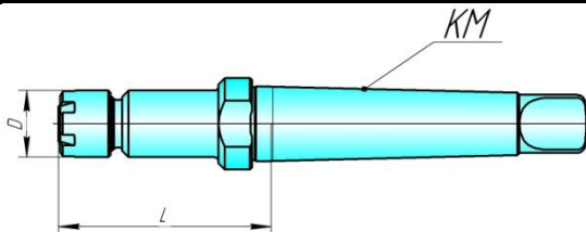
Цанговые патроны с хвостовиком Конус Морзе по ГОСТ 25557-2006 тип ВЕ (рис.1) и тип АЕ (рис.2)
